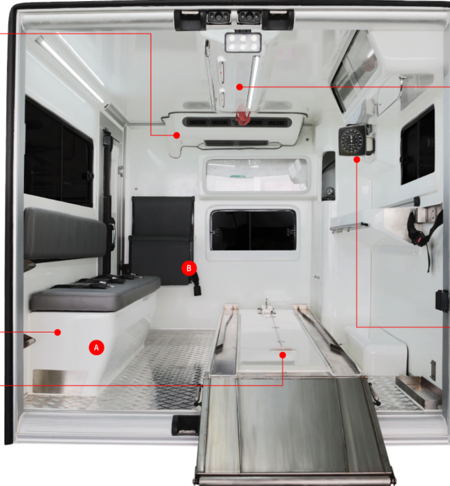
ที่เก็บสัมภาระขนาดใหญ่ 2 จุดพร้อมเคาน์เตอร์วางครุภัณฑ์ทางการแพทย์ เอนกประสงค์ 1 จุด สะดวกในการใช้สอย ผลิตจากไฟเบอร์กลาสชั้นเดียว
