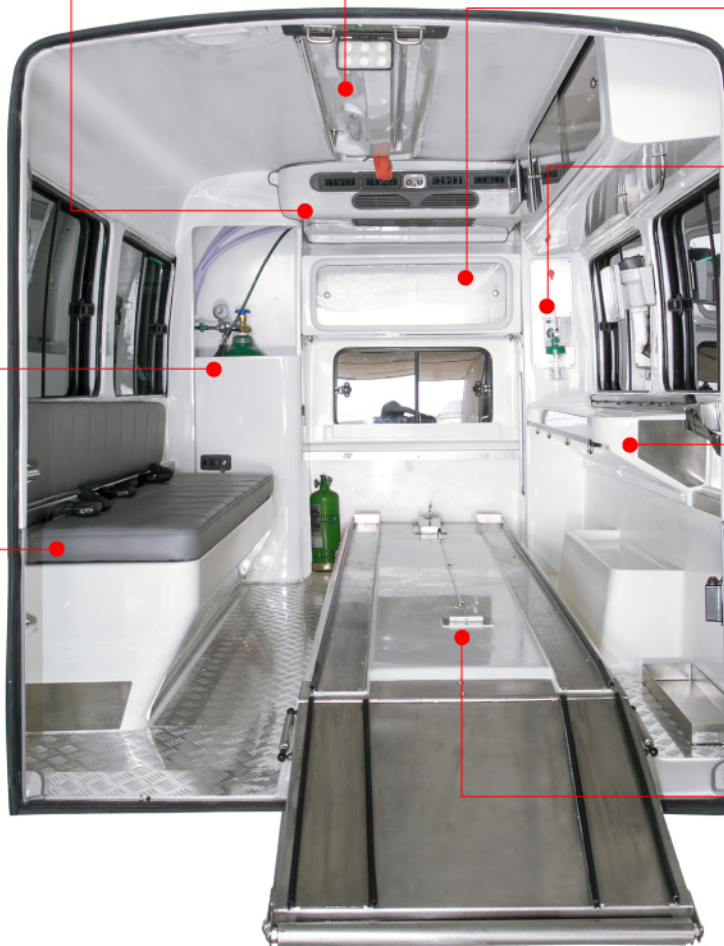
ชุดอุปกรณ์เพดานเอนกประสงค์ ที่แขวนน้ำเกลือ ไฟส่องสว่าง LED อายุการใช้งานยาวนาน พร้อมไฟสปอร์ตไลท์
